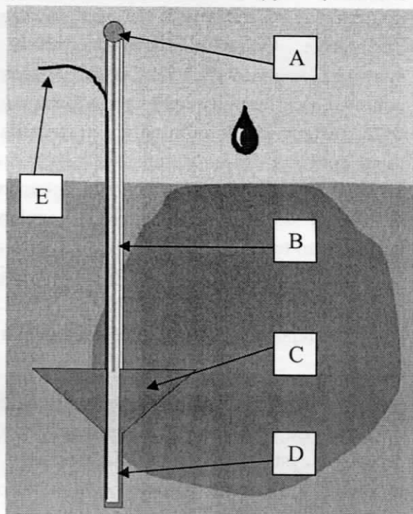
Rysunek 1. Sonda drenażu glebowego (SDG), A – wskaźnik poziomu, B – statyw, C – zbieracz, D – pływak, E – przewód polietylenowy
